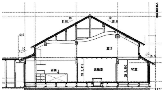
■今井町の家 断面図
